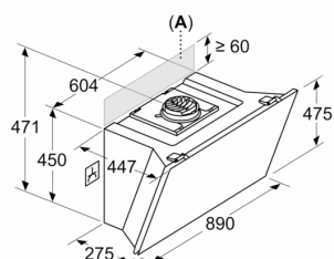
Измерване в mm Уред в режим циркулиращ въздух без димопровод
