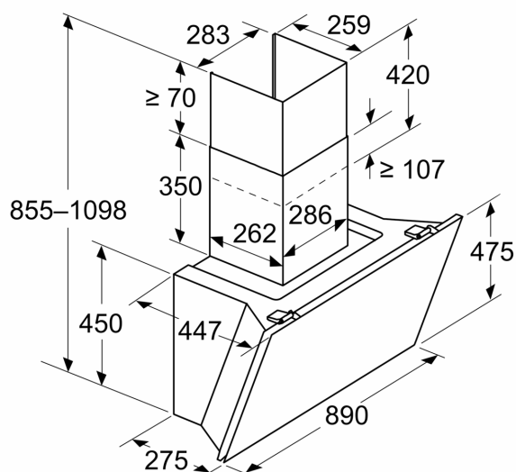
Измерване в mm Уред в режим отвеждане на въздуха
